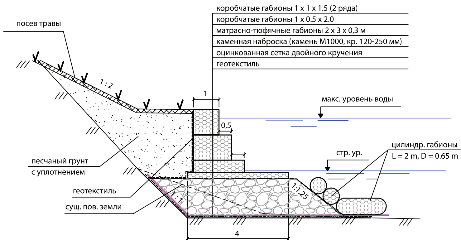
Объем основных работ на 100 м берегоукрепления
