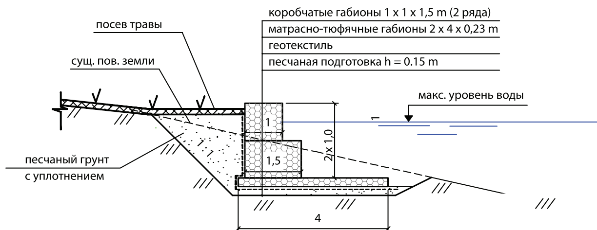
Объем основных работ на 100 м берегоукрепления
