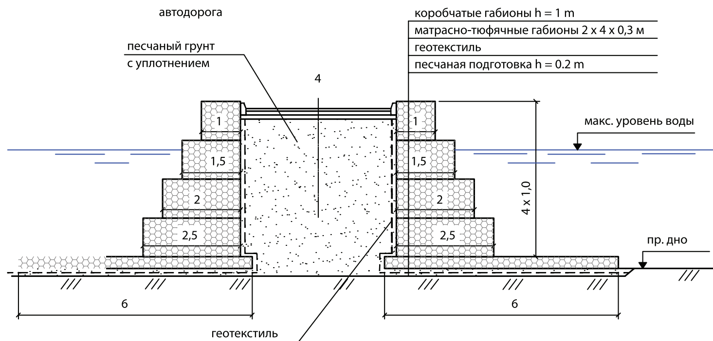
Объем основных работ на 10 м дамбы
